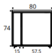
Pied double ruban vue de profil
